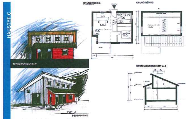
ABB. 4: HAUSTYP C M 1:200
