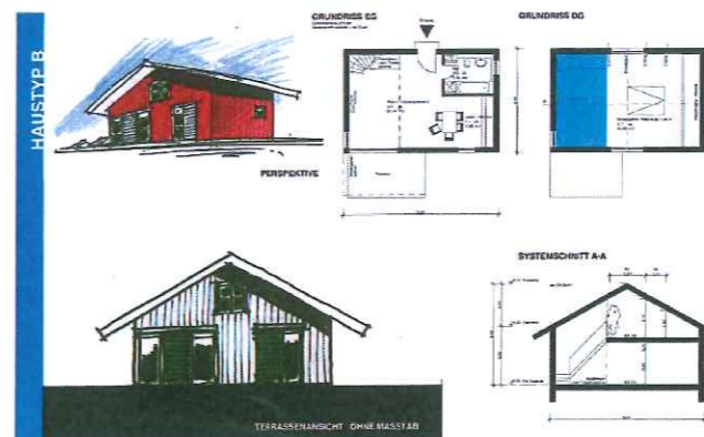
ABB. 3: HAUSTYP B M 1:200
