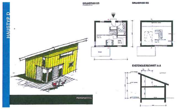
ABB. 5: HAUSTYP D M 1:200
