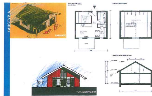
ABB. 2: HAUSTYP A M 1:200
